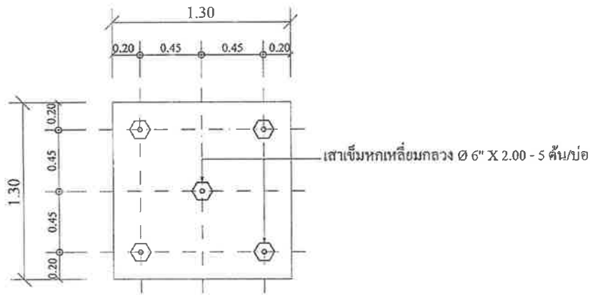
แปลนเสาเข็ม Scale 1:25
