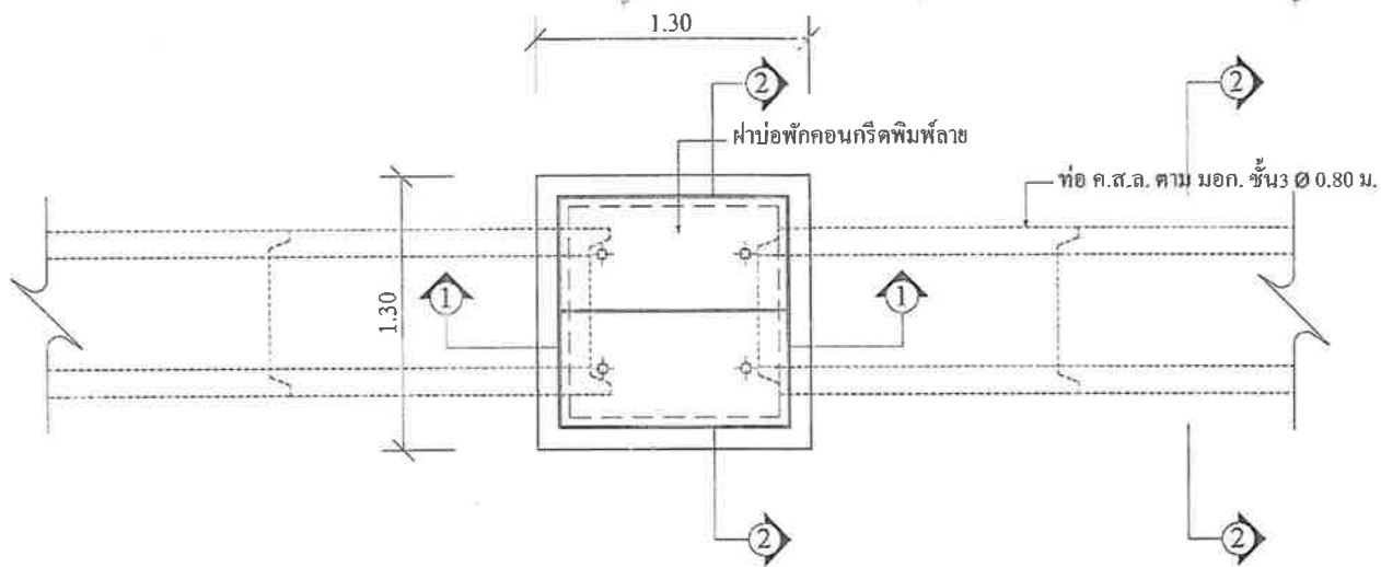
แปลนบ่อพัก Scale 1:25
