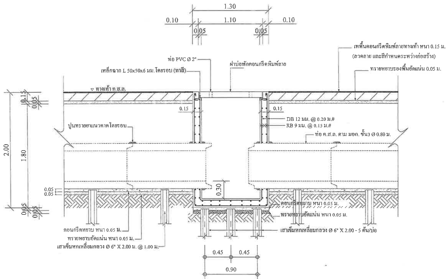
รูปตัด 1
