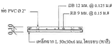
ขยายฝาบ่อพัก Scale 1:25
