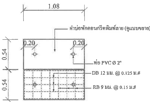
แปลนฝาบ่อพัก Scale 1:25
