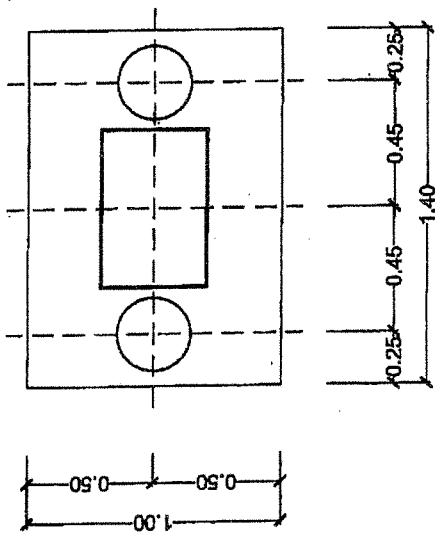
DETAIL F1 1:25
