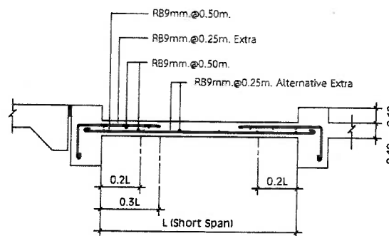
แบบขยายพื้น S1 มาตราส่วน 1:25
