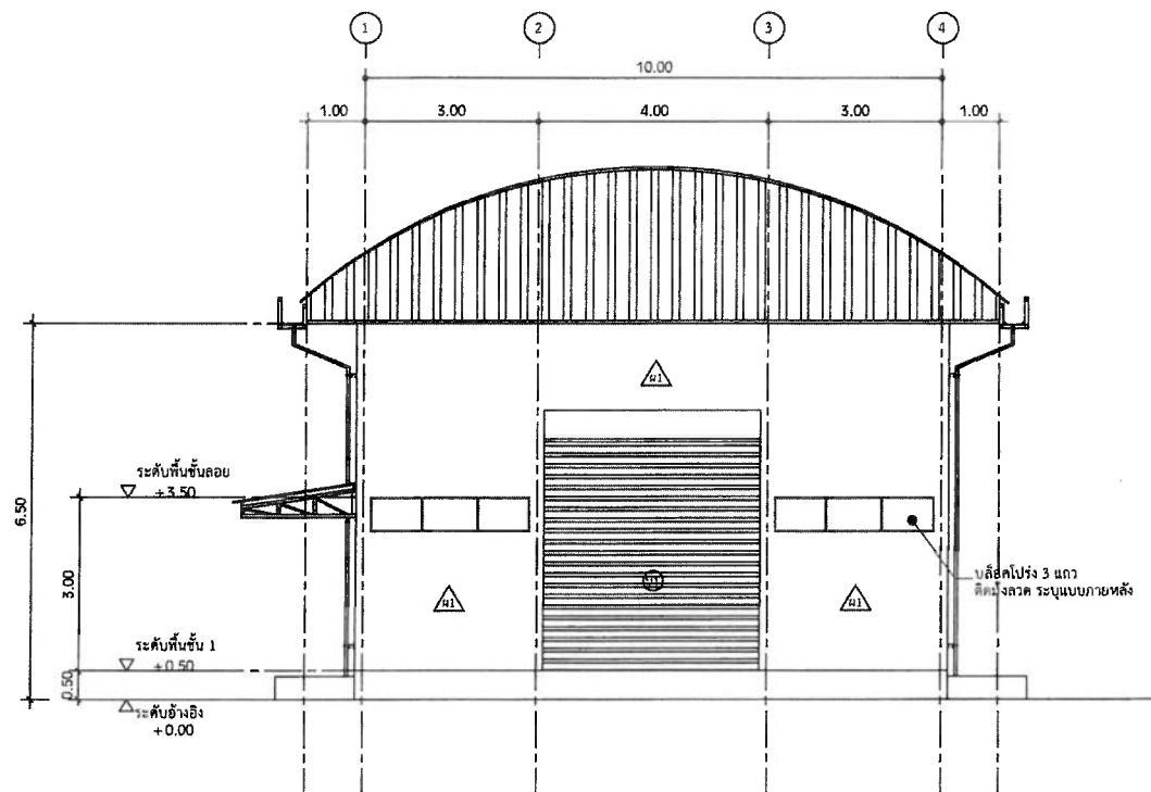
รูปด้าน 1 SCALE 1 100
