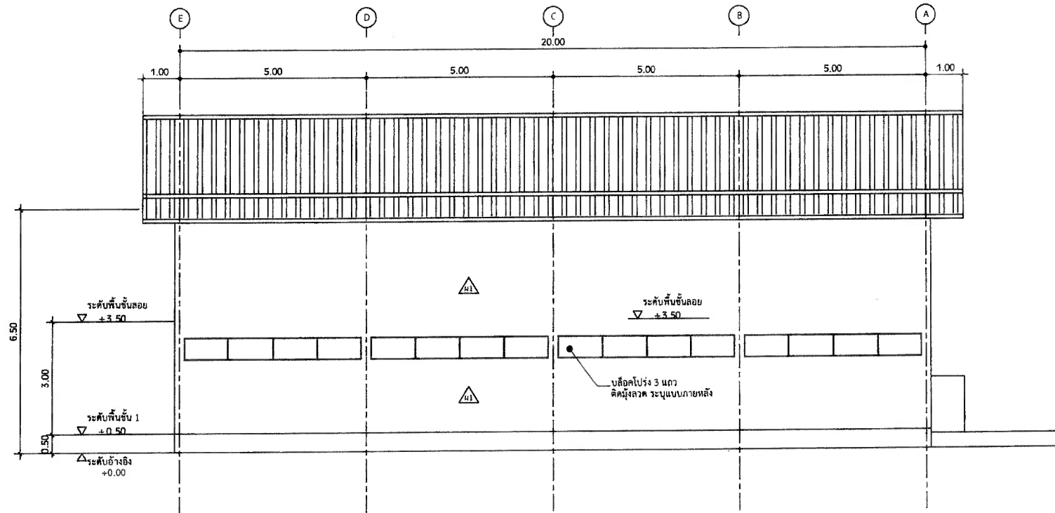
รูปด้าน 2 SCALE 1 : 100
