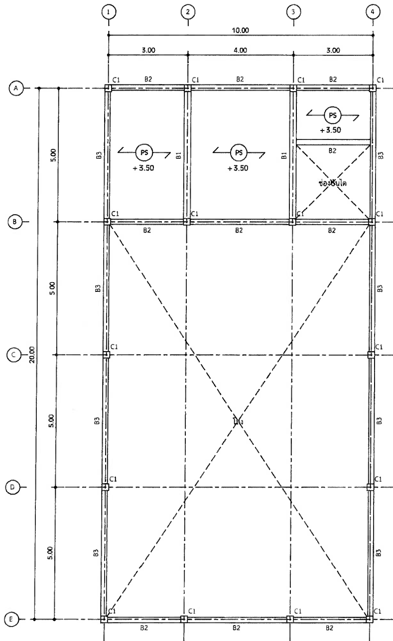
ผังเสา, คาน, พื้น ชั้นลอย SCALE 1 : 100
