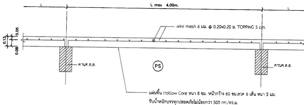
แบบขยายพื้น PS มาตราส่วน 1:25
