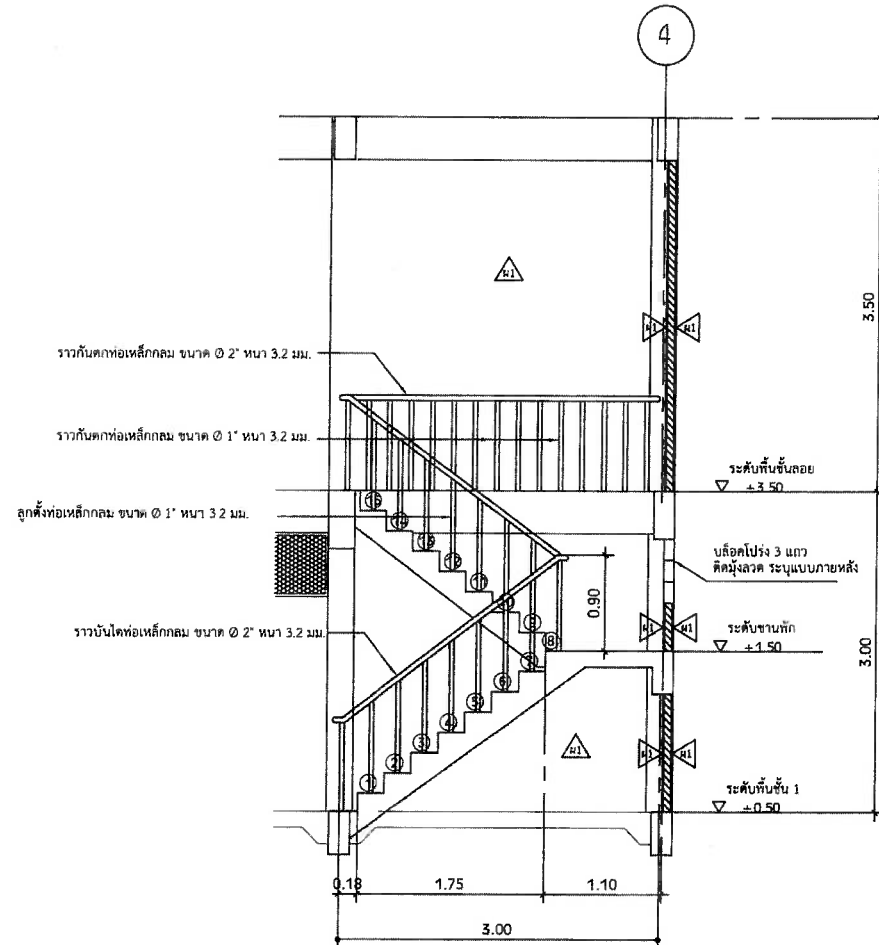
แบบขยายบันได ชั้นลอย SCALE 1 : 50
