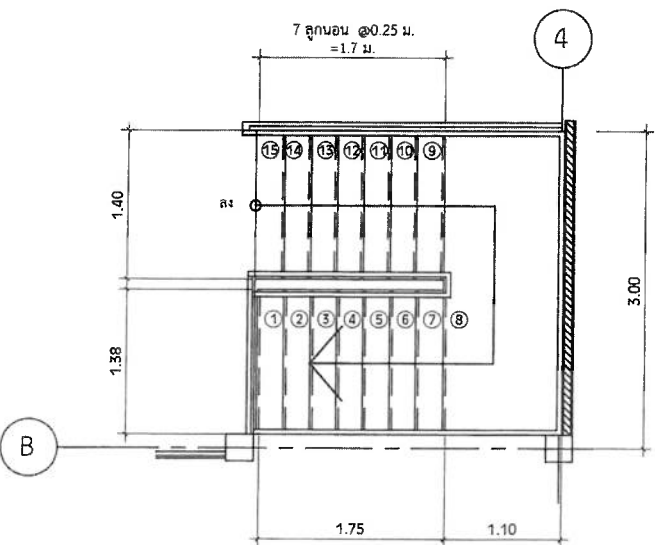
แบบขยายบันได ชั้นลอย SCALE 1 : 50
