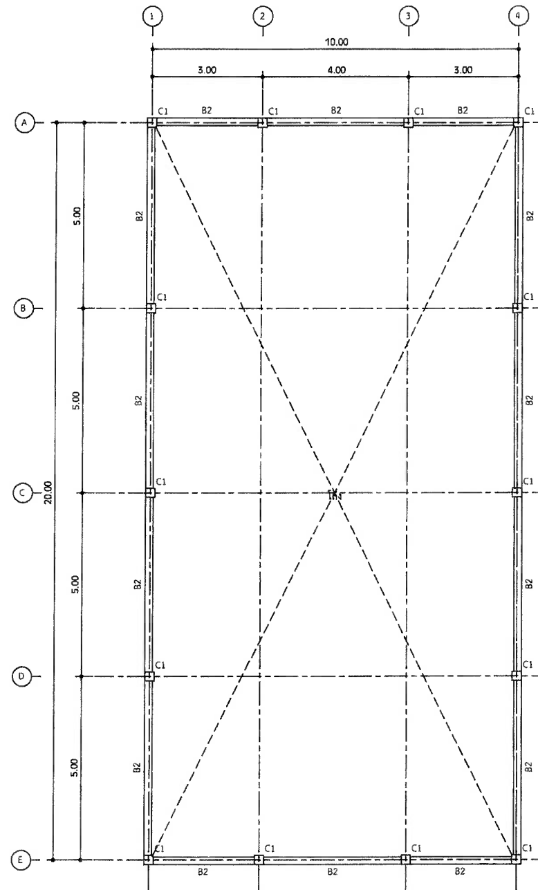
ผังคานชั้นอะเส SCALE 1 : 100
