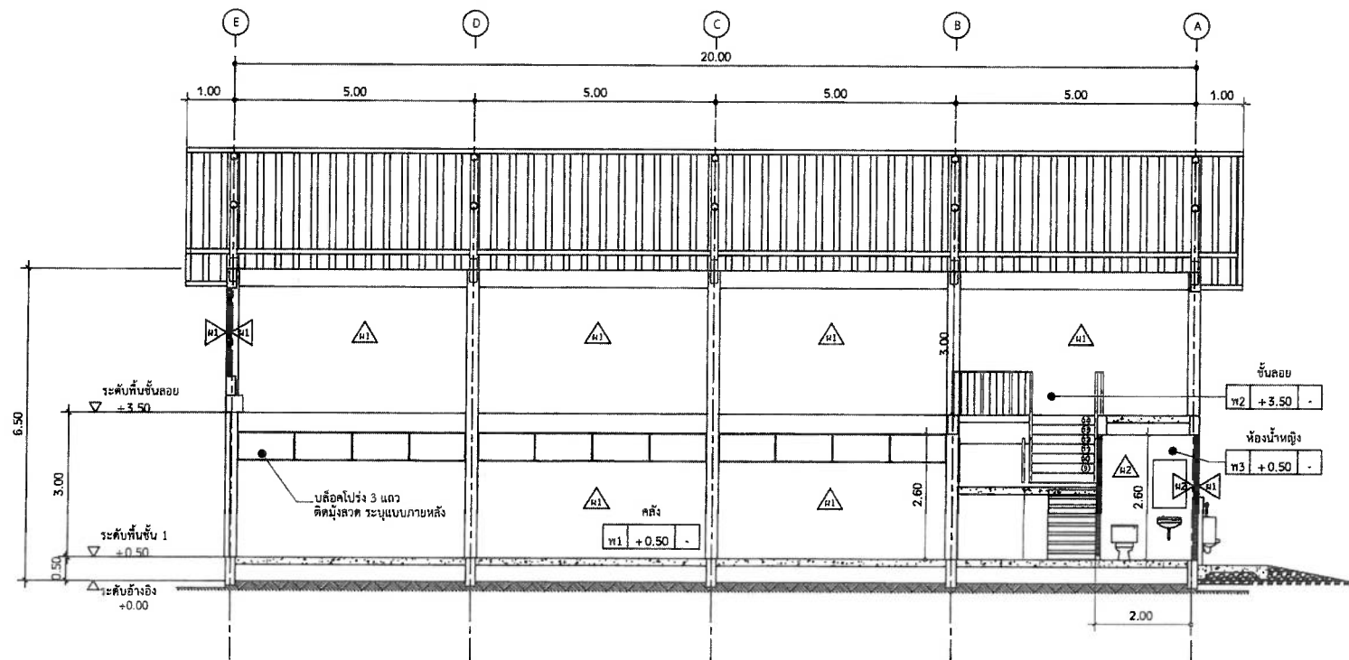
รูปตัด B SCALE 1 : 100
