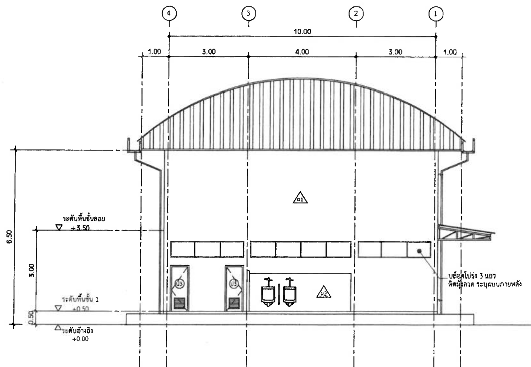
รูปด้าน 3
