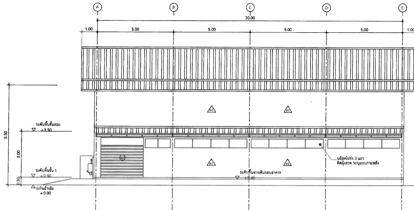
รูปด้าน 4 SCALE 1 : 100
