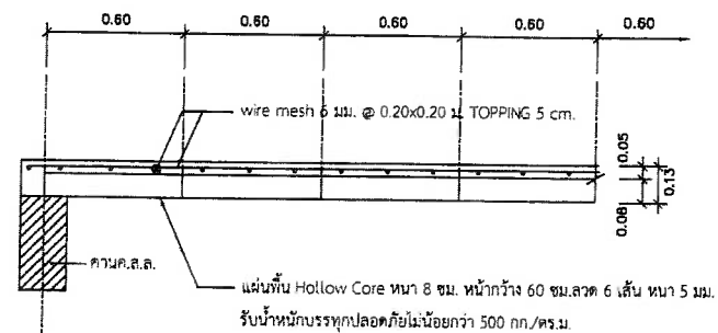
รูปตัดตามขวาง PS
