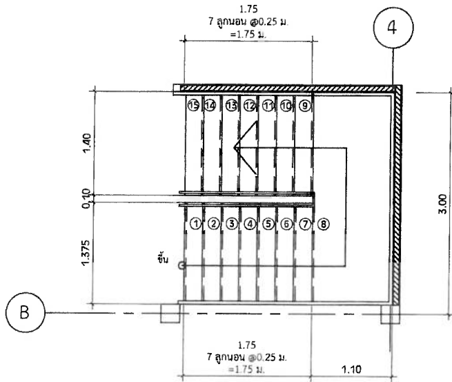
แบบขยายบันได ชั้น 1 SCALE 1 : 50
