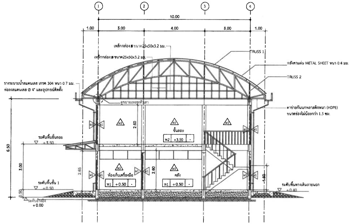
รูปตัด A SCALE 1 : 100
