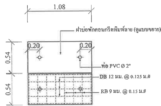
แปลนบ่อพัก
