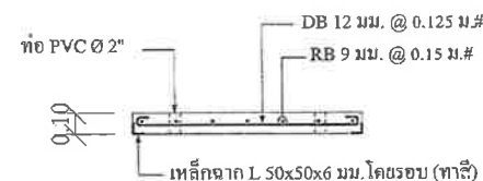
ขยายแปลนบ่อพัก
