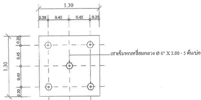
แปลนเสาเข็ม
