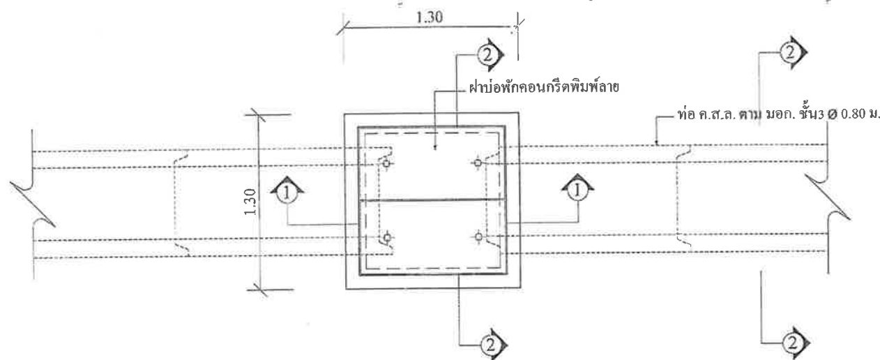
แปลนบ่อพัก
