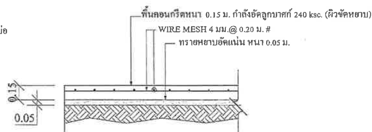
ขยายพื้นถนน ค.ส.ล.
