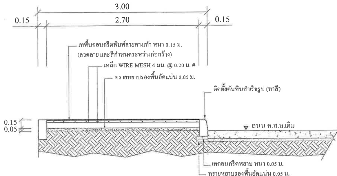
รูปตัด A
